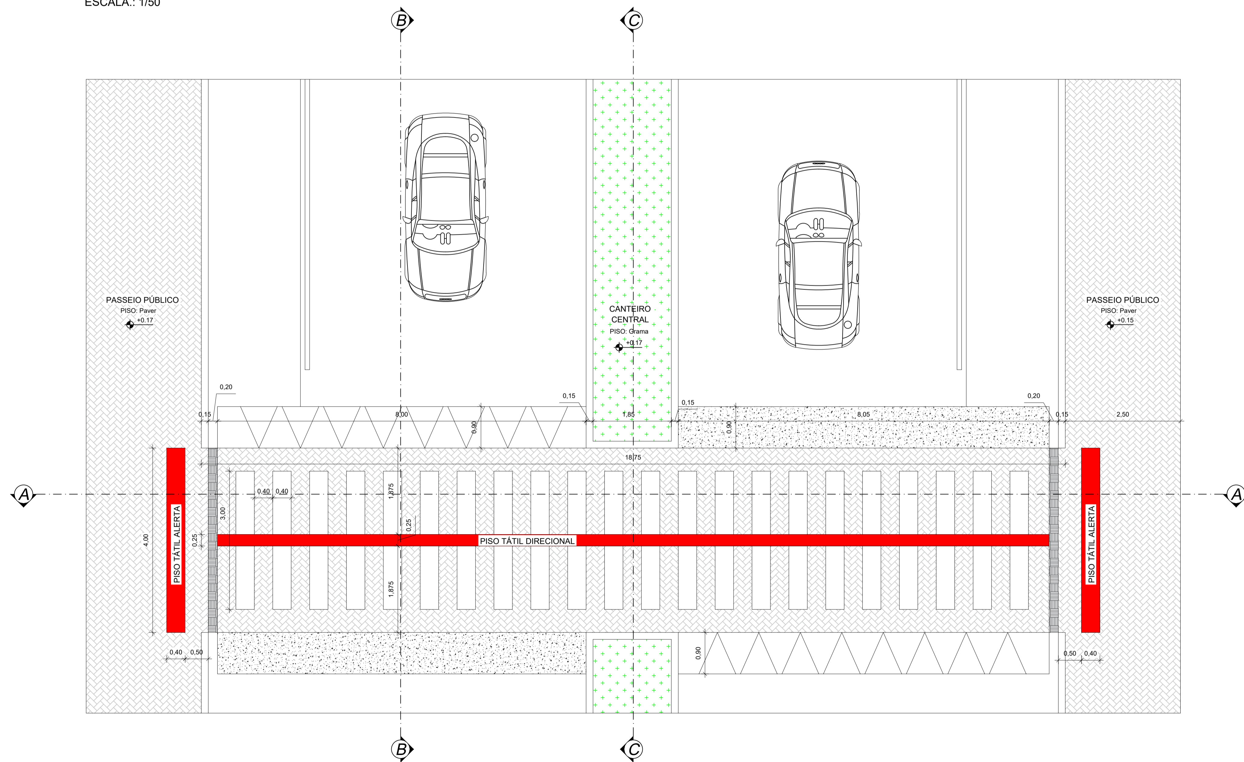
PASSEIO PÚBLICO AV. FLOR DO SERTÃO ESQ. RUA AFONSO CENEDESSE QUADRA.: 11 E 12 ESCALA.: 1/50
